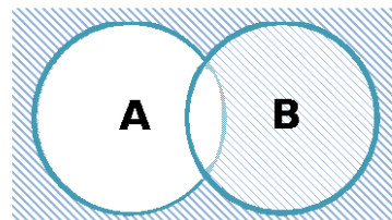
(A \square) = U - A
