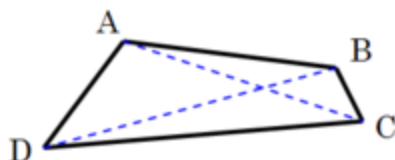
Un cuadrilátero con sus diagonales.
